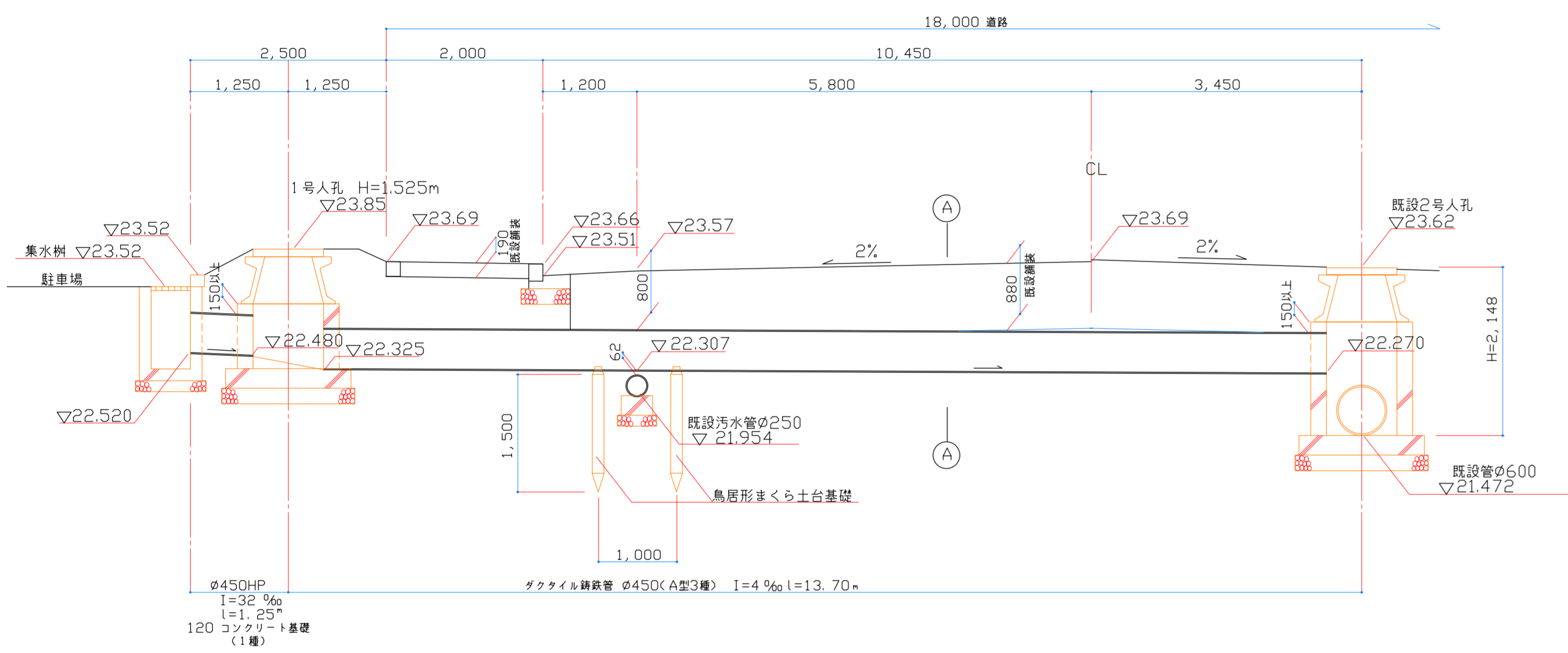
① 縦断図 S=1:50
